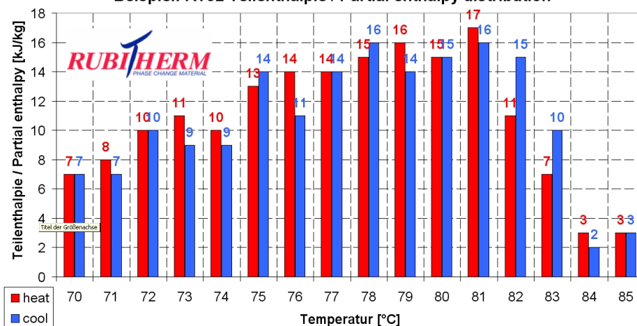
Beispiel: RT82 Teilenthalpie / Partial enthalpy distribution
