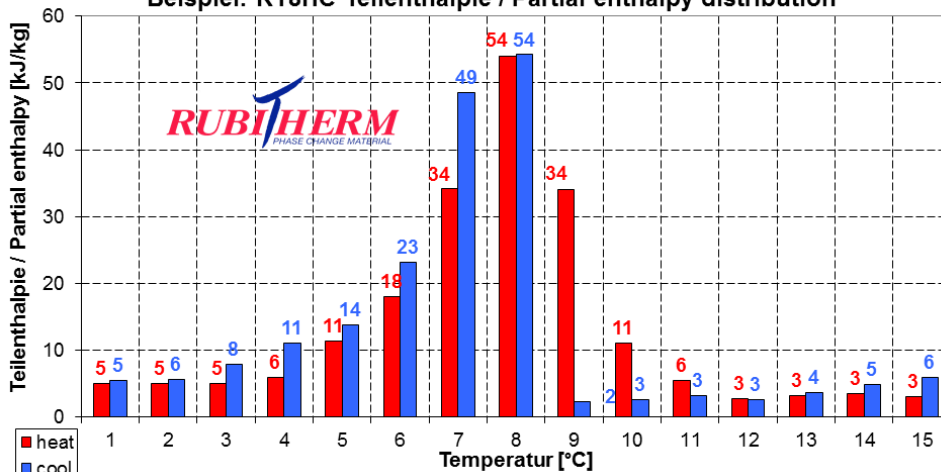
Beispiel: RT8HC Teilenthalpie / Partial enthalpy distribution
