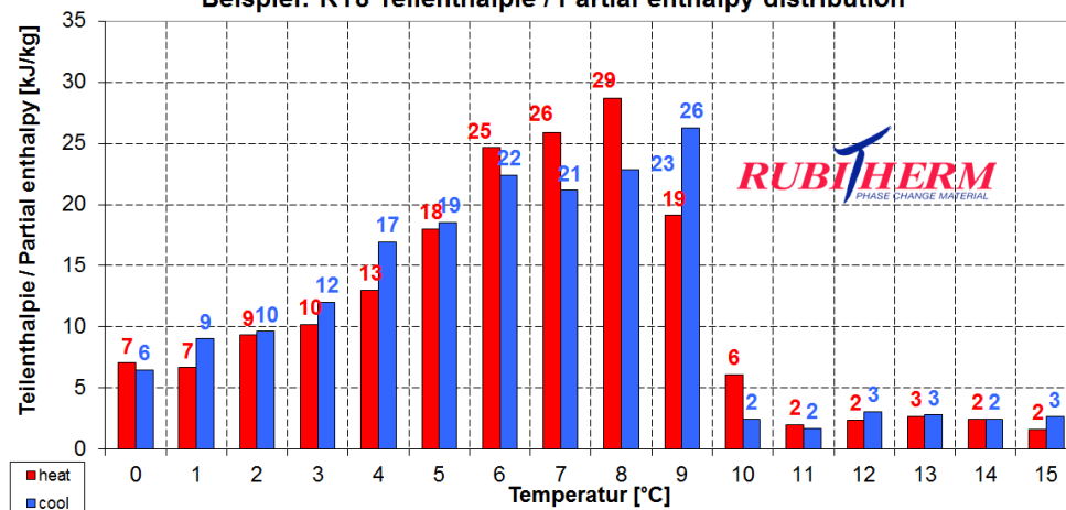
Beispiel: RT8 Teilenthalpie / Partial enthalpy distribution
