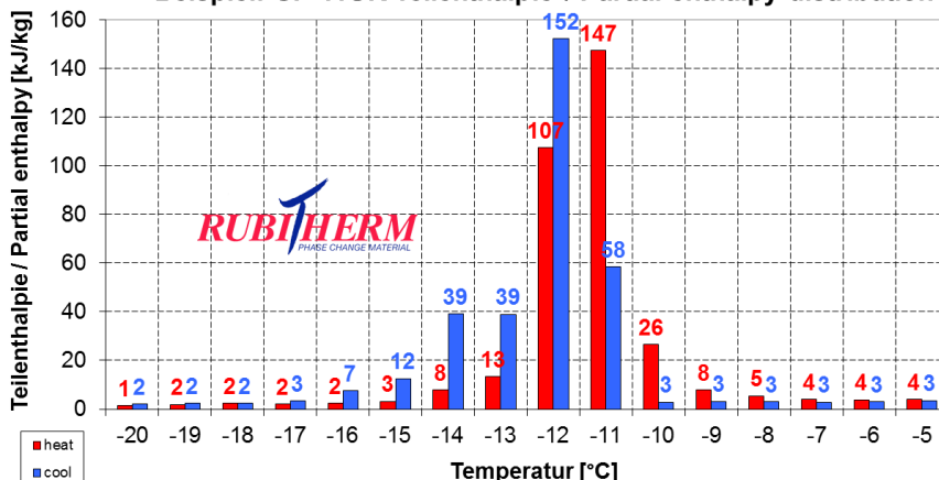
Beispiel: SP-11UK Teilenthalpie / Partial enthalpy distribution
