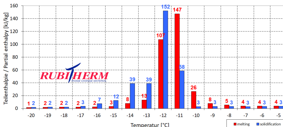
Beispiel / example: SP-11UK Teilenthalpie / Partial enthalpy distribution*
