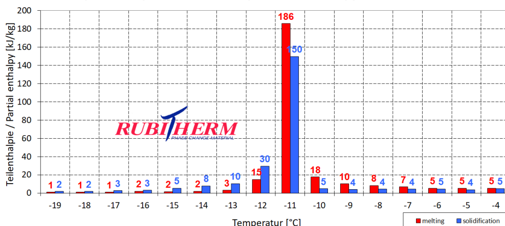
Beispiel / example: SP-11 Teilenthalpie / Partial enthalpy distribution*
