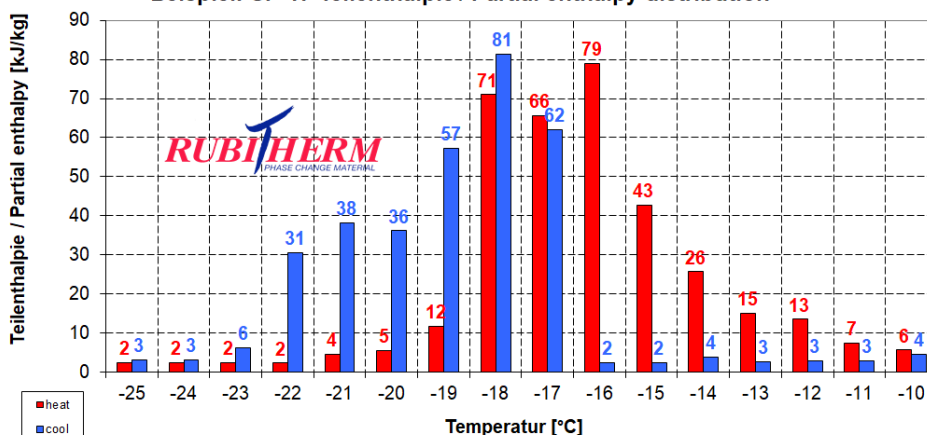
Beispiel: SP-17 Teilenthalpie / Partial enthalpy distribution
