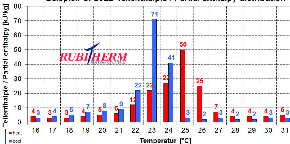
Beispiel: SP25E2 Teilenthalpie / Partial enthalpy distribution
