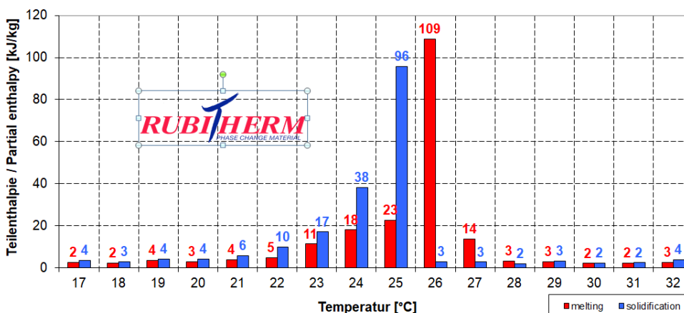
Beispiel / example: SP26E Teilenthalpie / Partial enthalpy distribution*
