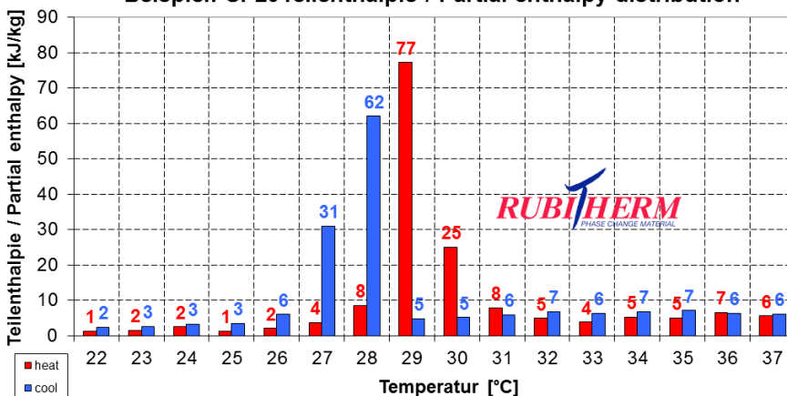
Beispiel: SP29 Teilenthalpie / Partial enthalpy distribution
