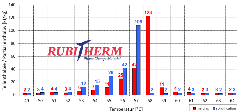
Beispiel / example: SP58_gel Teilenthalpie / Partial enthalpy distribution*
