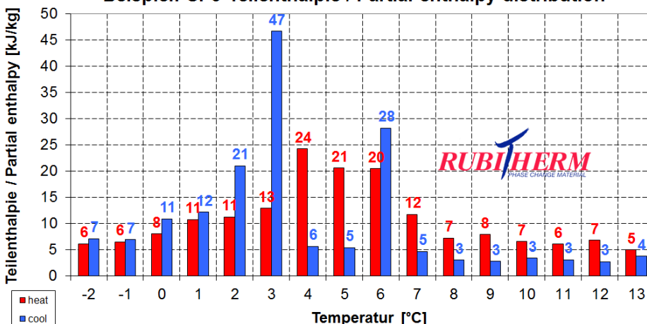
Beispiel: SP5 Teilenthalpie / Partial enthalpy distribution
