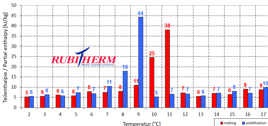
Beispiel / example: SP9_gel Teilenthalpie / Partial enthalpy distribution*
